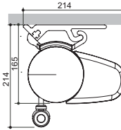
Deckenmontage
