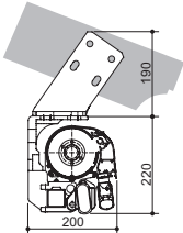
Dachsparrenmontage
