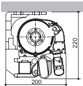
Deckenmontage
