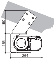
Dachsparrenmontage
