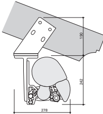
Dachsparrenmontage
