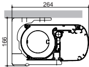
Deckenmontage
