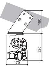
Dachsparrenmontage
